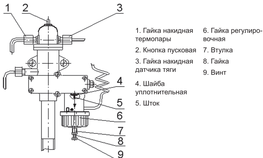
Рисунок 2. Блок автоматики
